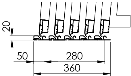
DETAIL A Maßstab 1 : 10
