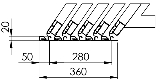
DETAIL A Maßstab 1 : 10
